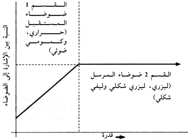
الشكل 2-35 رسم بياني لنسبة الإشارة إلى قدرة الضوء بالمقارنة مع الطاقة عند خرج جهاز الاستقبال البصري.
